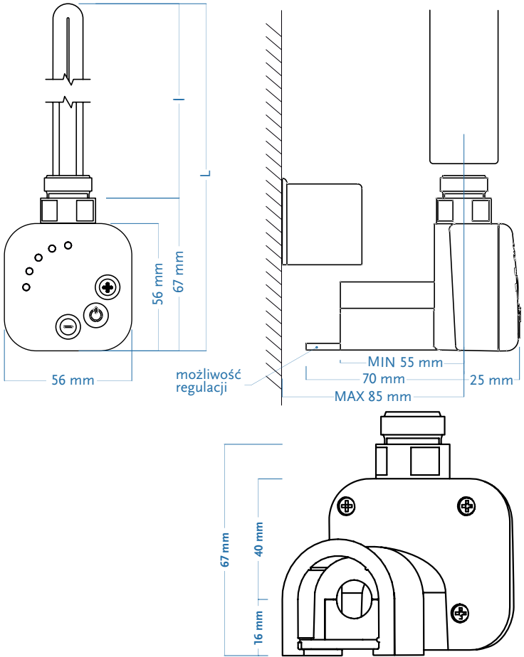
GKM - schemat grzałki
