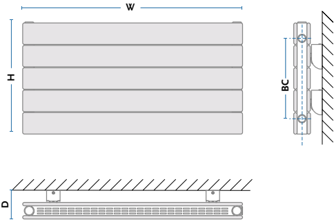
[31] / [32] - podłączenie 180°
