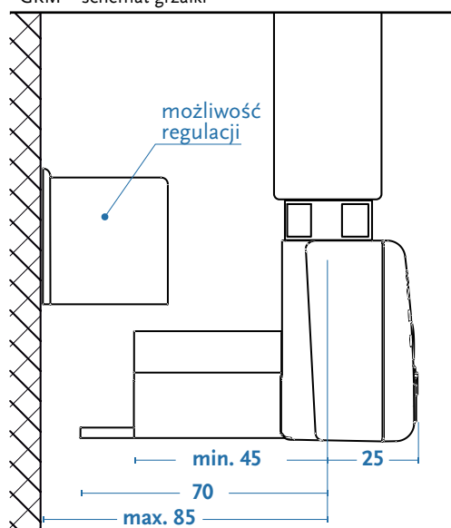
GKM - schemat grzałki
