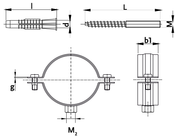
USZ 75 - USZ 220
